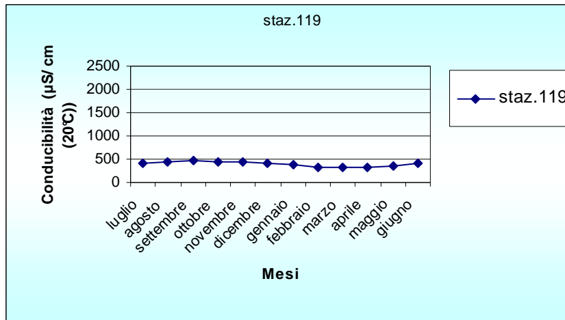
Figura 3.1.3 – Andamento medio mensile della conducibilità elettrica nella stazione Fiumedinisi 119
