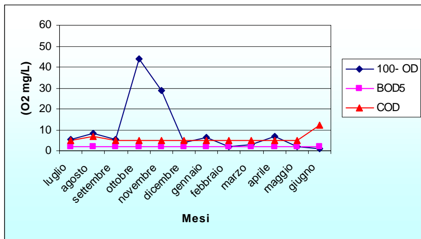
Figura 3.1.5 – Andamento medio mensile della concentrazione di ossigeno disciolto, BOD, COD nella stazione Fiumedinisi 119
