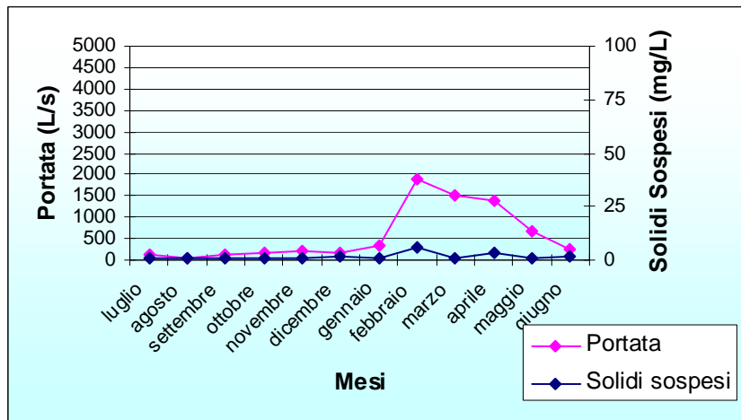
Figura 3.1.4 – Andamento medio mensile della portata e della concentrazione dei solidi sospesi nella stazione Fiumedinisi 119
